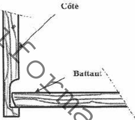
Détail montage battant
